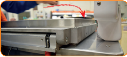
Étape 6 : Refermer le cadre de grille sur la machine
